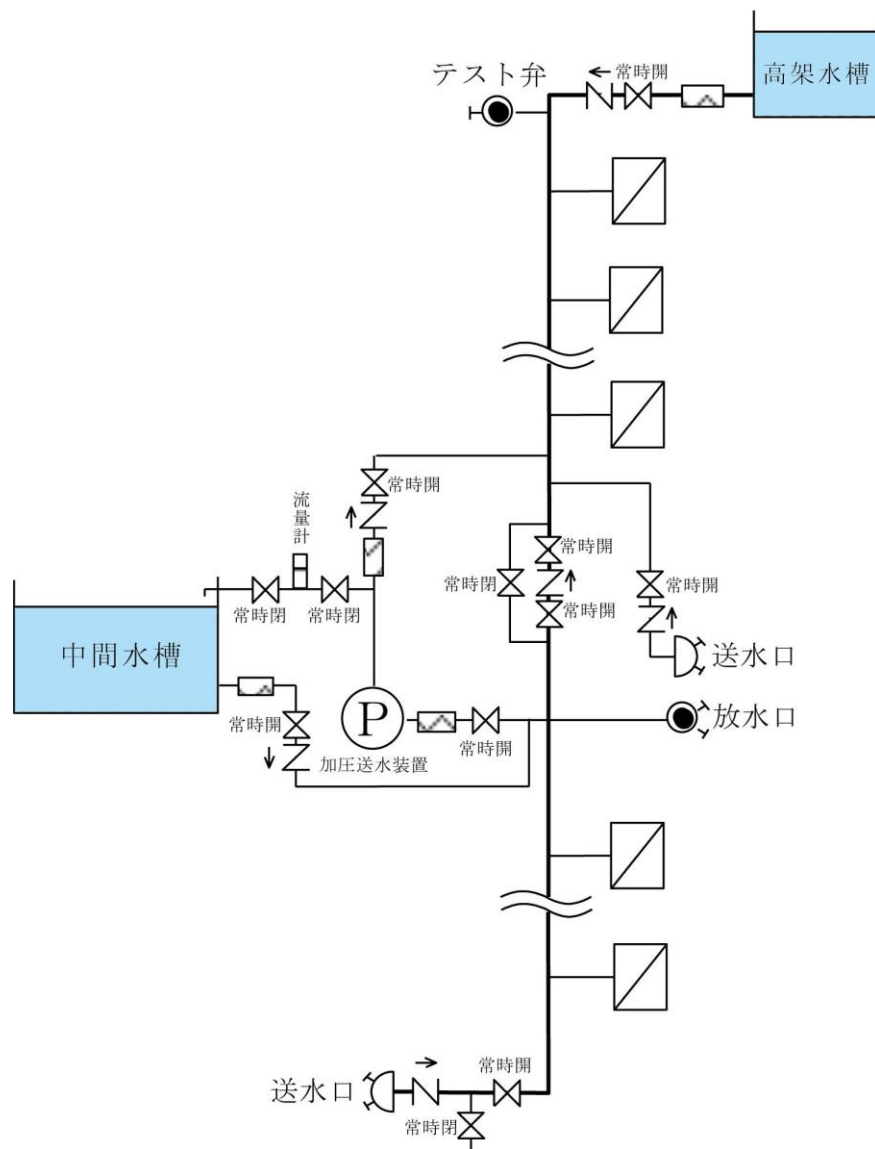
第20-2図 加圧送水装置を設けた場合の配管例
