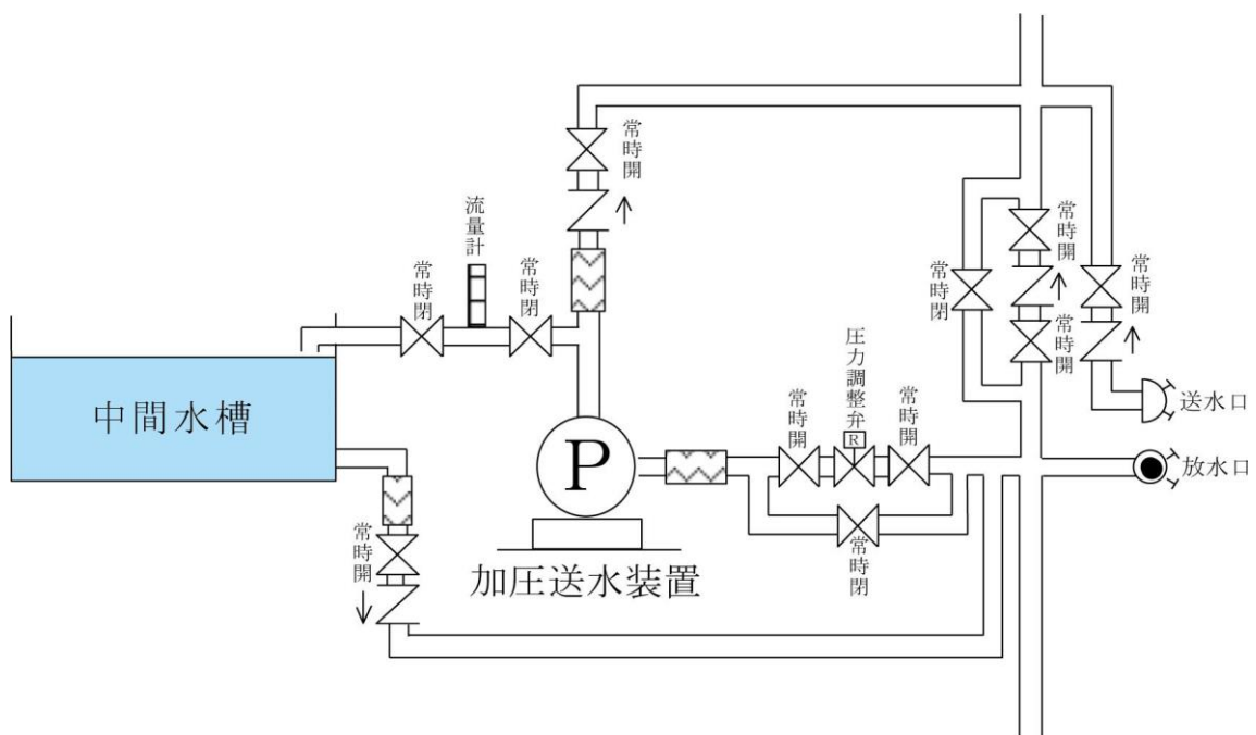
第20-3図b 圧力調整弁を設置した場合
