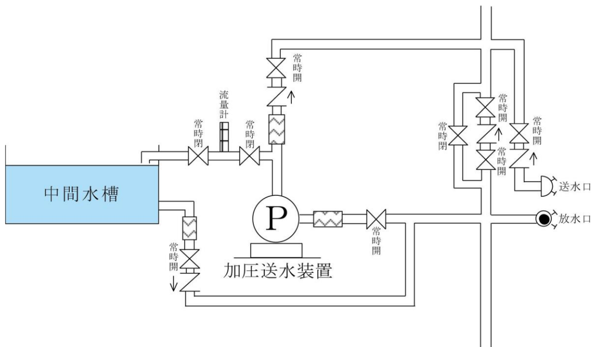
第20-3図a 圧力調整弁を設置しない場合
