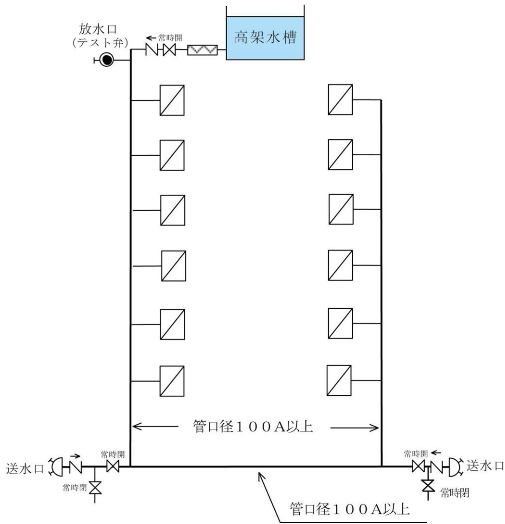
第20－1図 連結送水管の配管例
