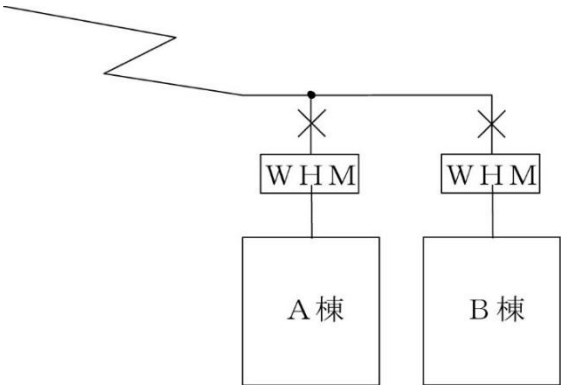
引込線の接続と引込口配線の関係
