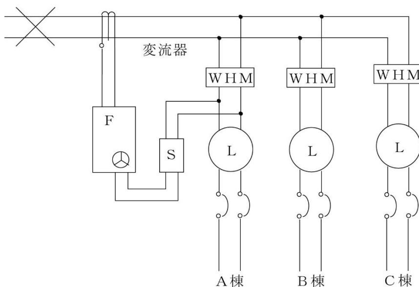
変流器の設置位置と電路との関係
